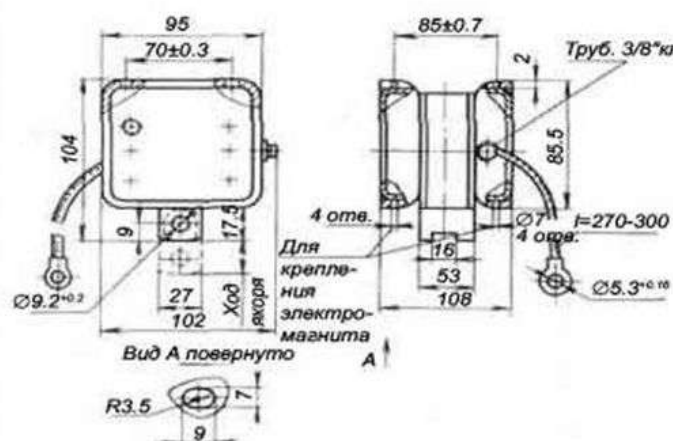
МИС 5-го габарита тянущего исполнения
