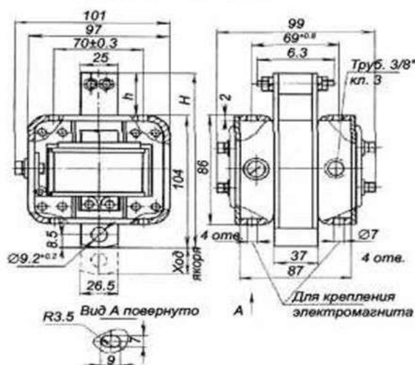
1 1, 2, 3, 4 габариты тянущего исполнения
