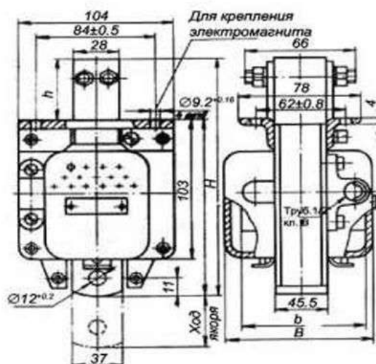
МИС 6-го габарита толкающего исполнения
