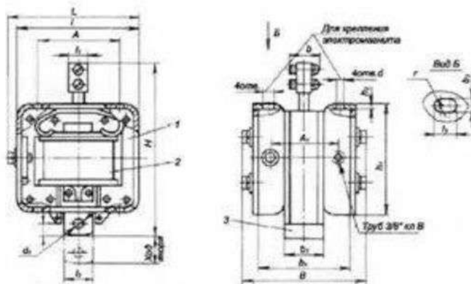
1, 2, 3 габариты толкающего исполнения
