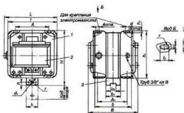
1 1, 2, 3, 4 габариты тянущего исполнения
