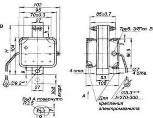
МИС 5-го габарита толкающего исполнения
